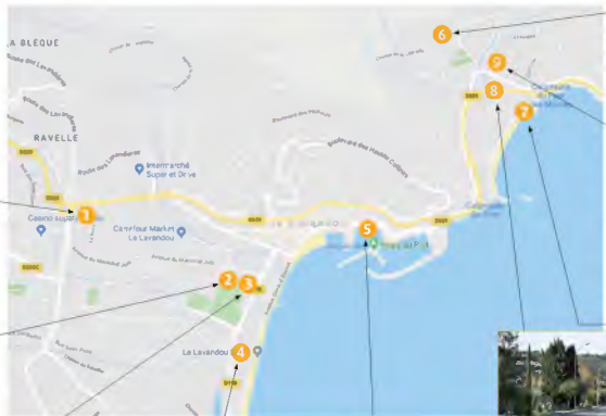
Création de passages surélevés sur la route départementale. Travaux réalisés par le Conseil départemental.
